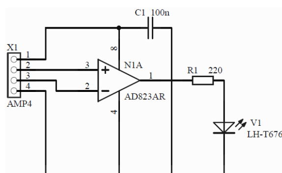
Abbildung 1 Beispielschaltung
