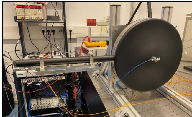
Versuchsaufbau für Reaktionsräder im ESTEC-Labor
